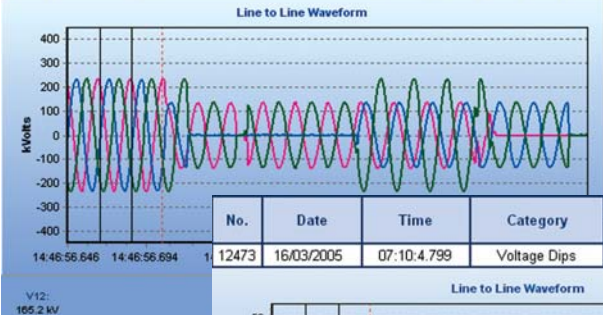
VOLTAGE SAG
