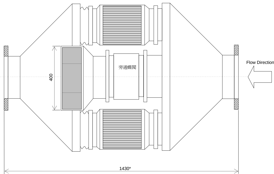
正視圖
