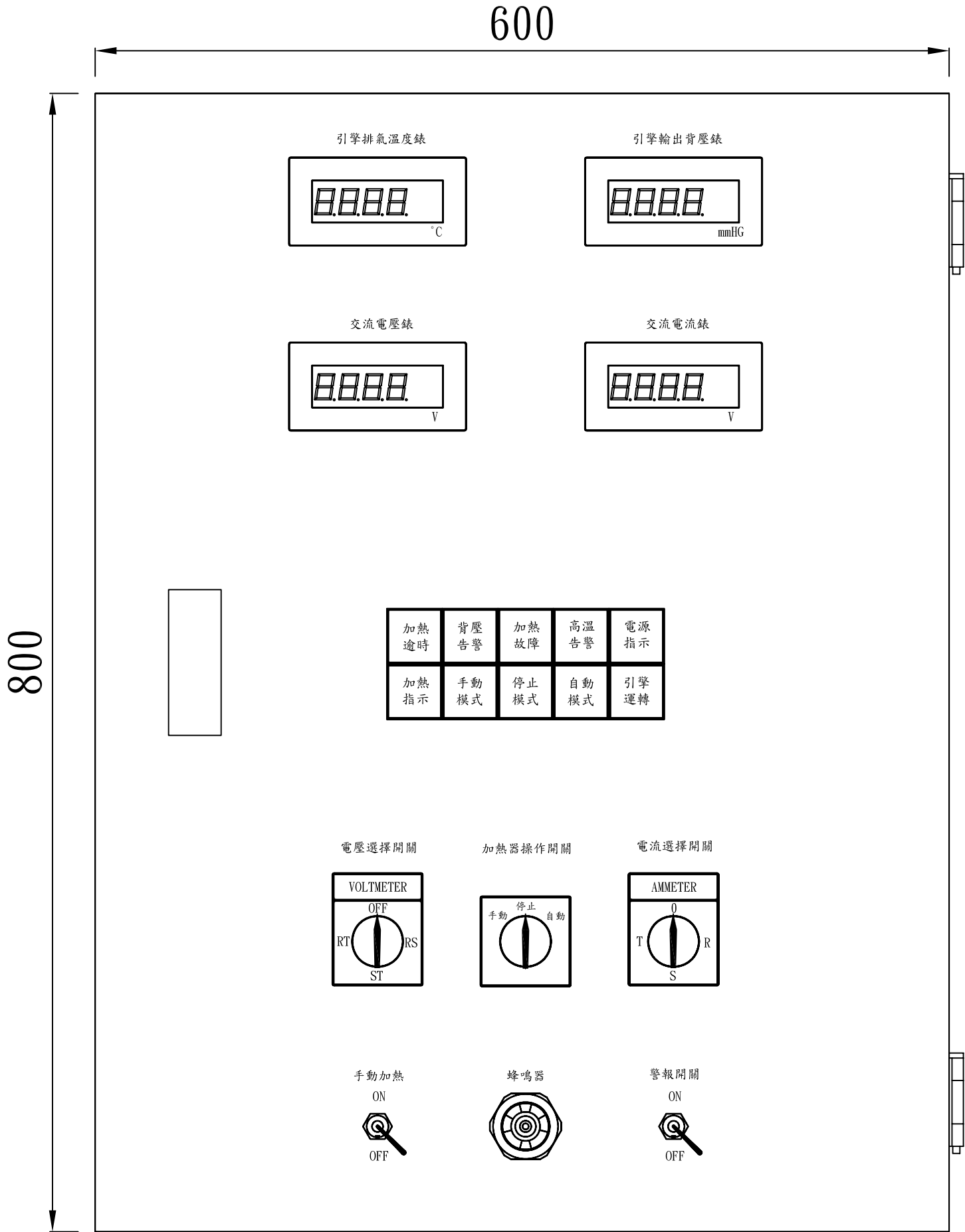
正視圖
