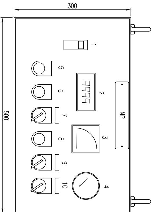
正視圖
